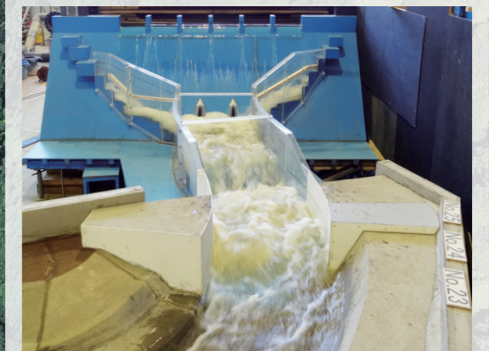
水理模型実験の様子
