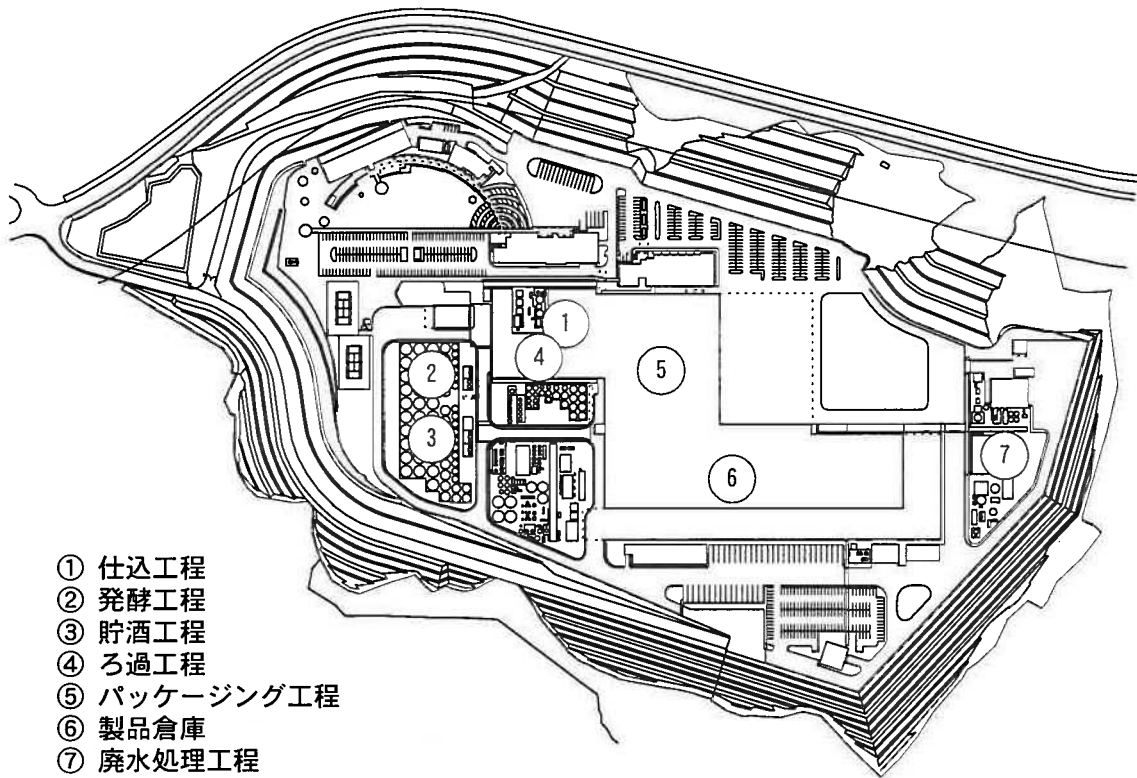
3 工場配置図
