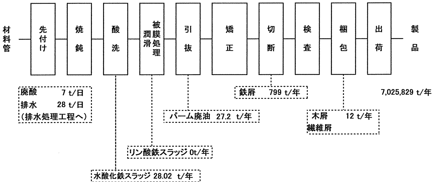
図1 冷間引抜鋼管製造フローシート
