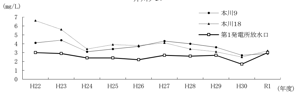
芹川ダム
