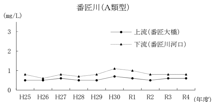
図 i 番匠川水系 BOD 年間平均値の経年変化
