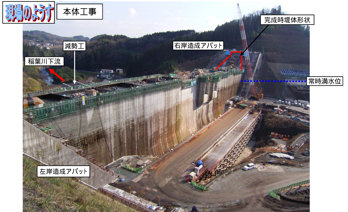
堤体コンクリート全体数量約22万m 3 のうち、12月末で約20万m 3 のコンクリート打設が完了します。
