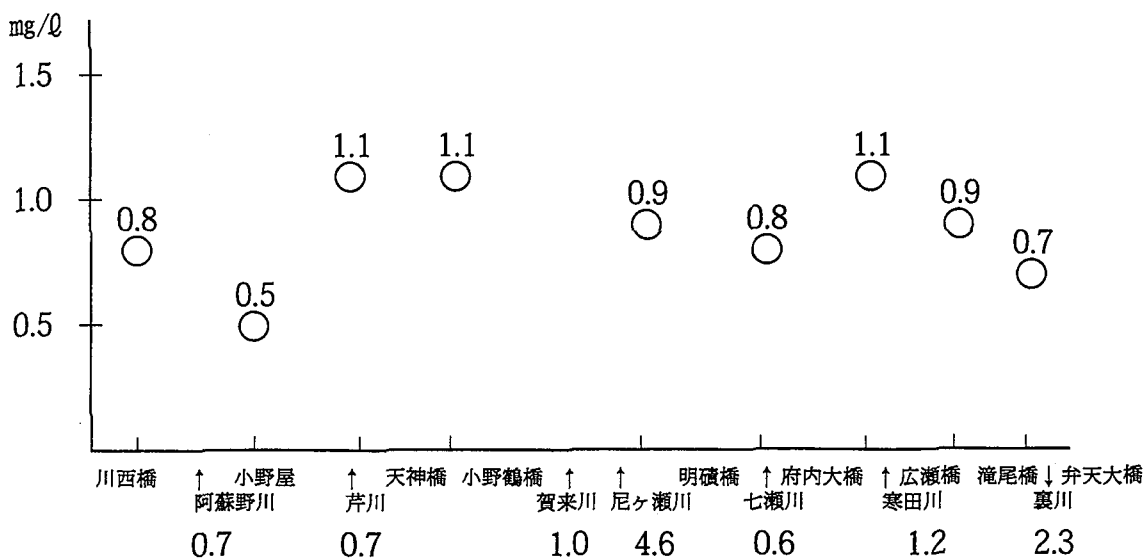
図2-7 大分川水系水質縦断変化（BOD年平均値）
